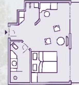
Beispiel Zimmer und Raumschnitt
